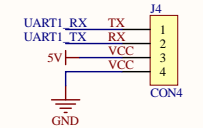
蓝牙模块
